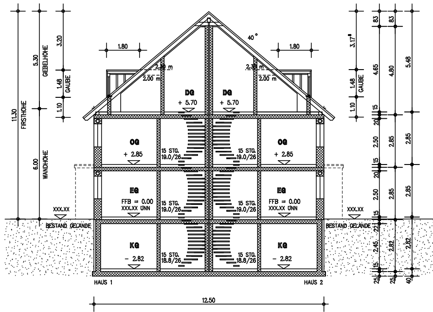
SCHNITT A 12 - A 12
