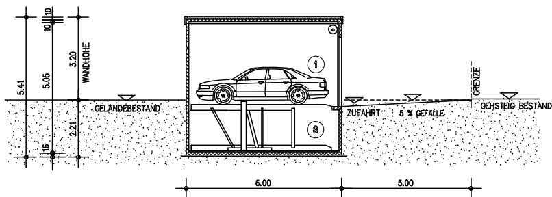
SCHNITT DUPLEXGARAGE B 11 - B 11
