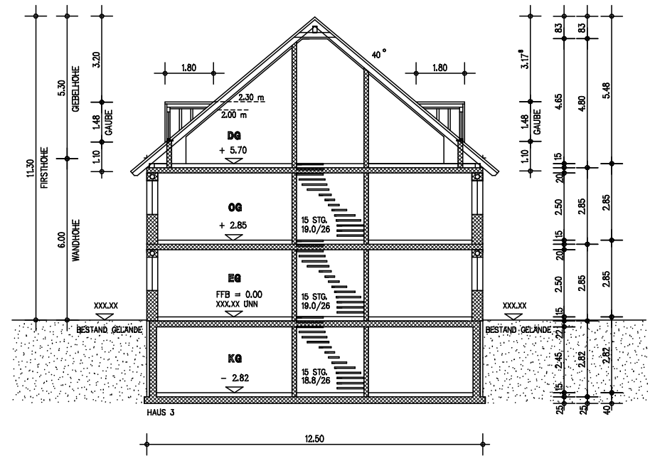
SCHNITT A 11 - A 11
