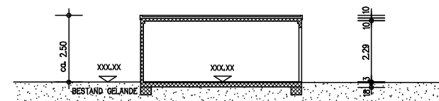
SCHNITT EINZELGARAGE B 12 - B 12
