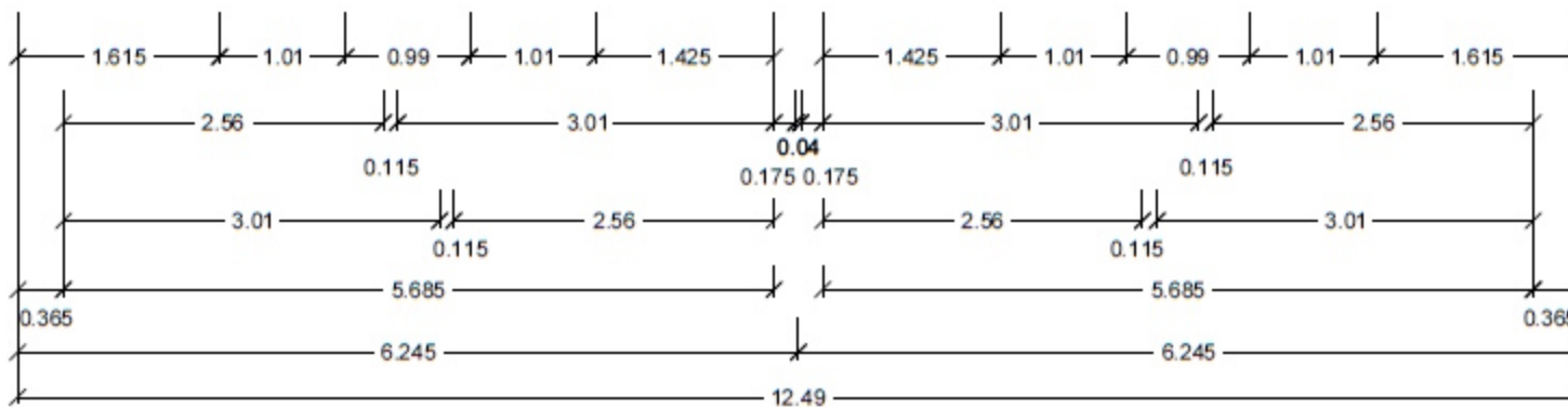
Grundriss OG
